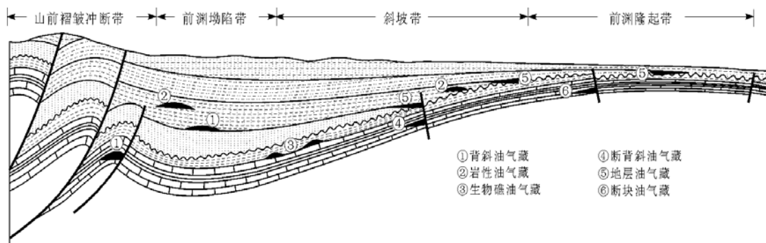
图2 从造山带到盆地不同构造带油气藏类型分布 [24]
