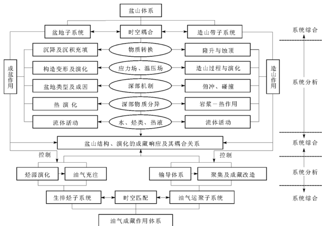
图 1 盆山体系与油气成藏作用体系综合研究框架 [21]
