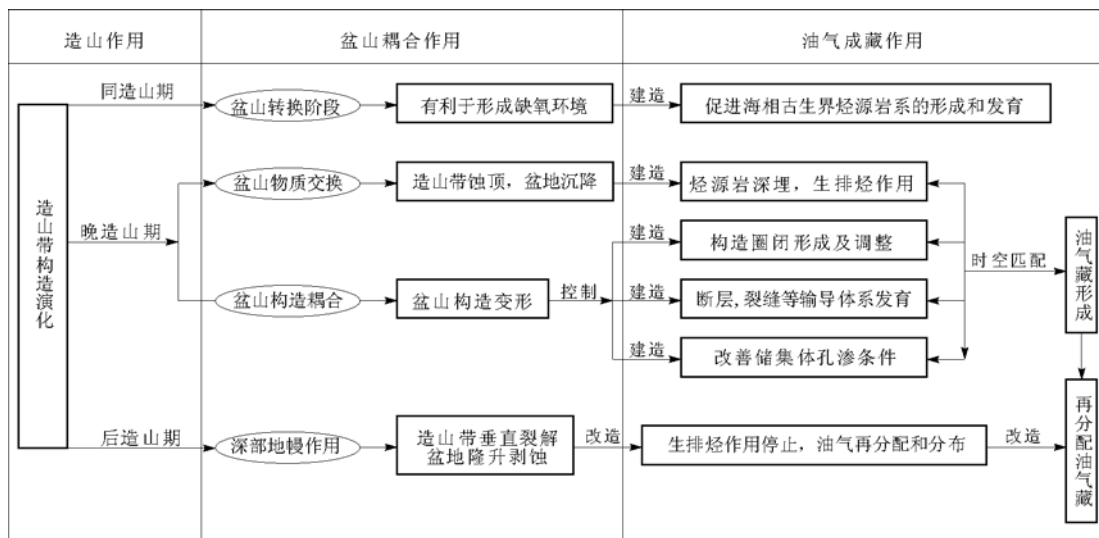
图 3 盆山体系演化与油气成藏作用相互关系模型
