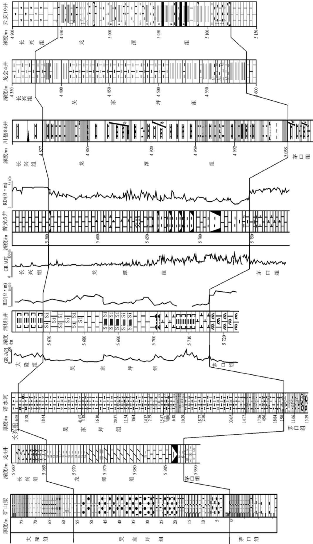
图4 川东北地区龙潭组地层横向对比剖面位置见图1。
