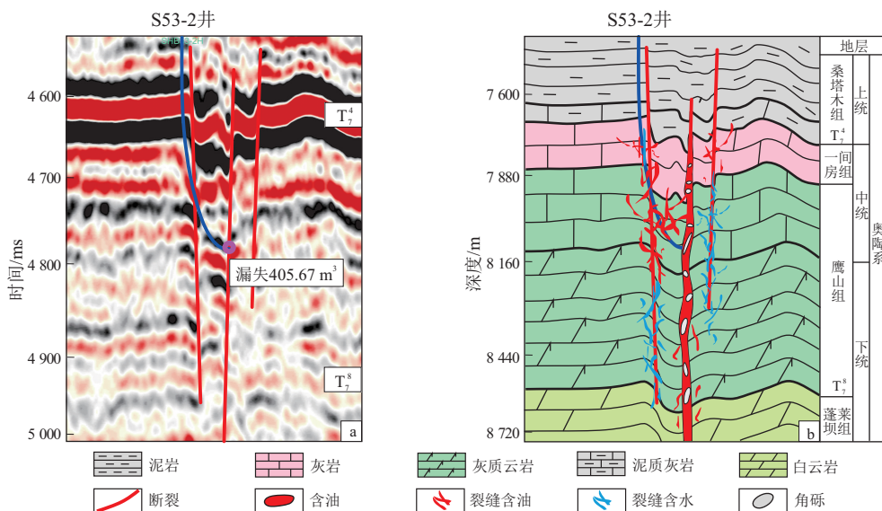
图2 塔里木盆地顺北地区S53-2井剖面特征
