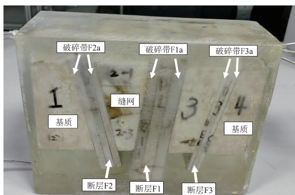
图 7 塔里木盆地顺北地区 S53-2 井实验模型
